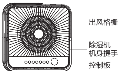
顶面
