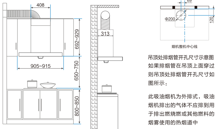
排烟管走橱柜安装示意图
