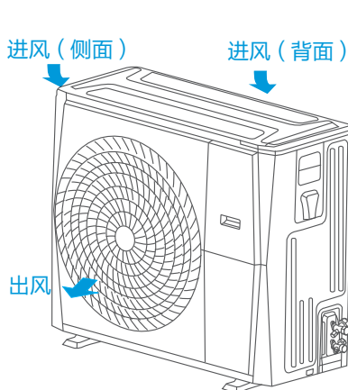
单风轮80/100/120/140外机
