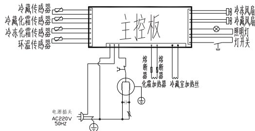
运行电容C*为可选件(根据压缩机选配) 电气原理图
