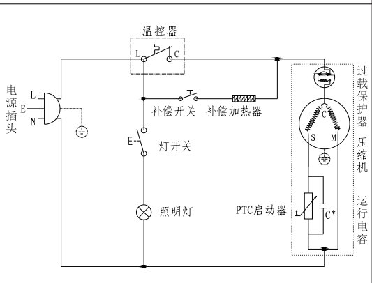
运行电容C*为可选件(根据压缩机选配) 电气原理图
