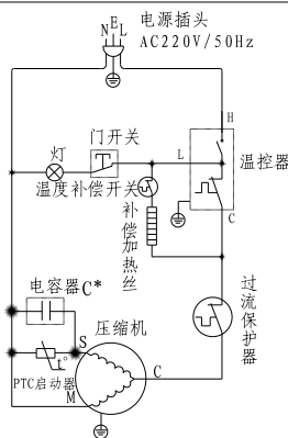
运行电容C*为可选件(根据压缩机选配)电气原理图
