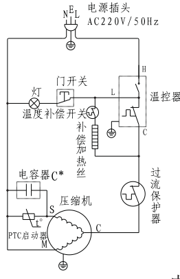
运行电容C*为可选项(根据压缩机选配)电气原理图
