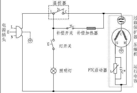
运行电容C*为可选件(根据压缩机选配) 电气原理图
