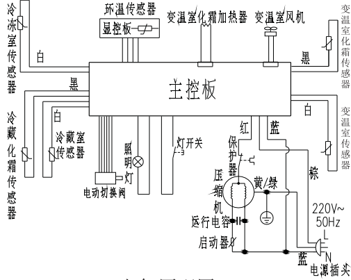
电气原理图
