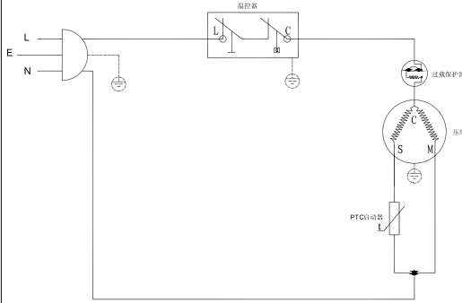
电气原理图
