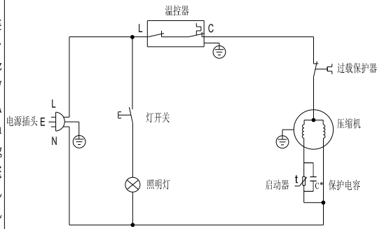
运行电容C*为可选件(根据压缩机选配) 电气原理图
