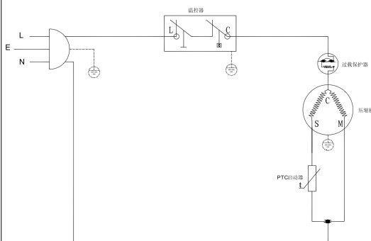
电气原理图
