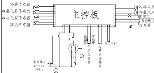
运行电容C*为可选件(根据压缩机选配) 电气原理图
