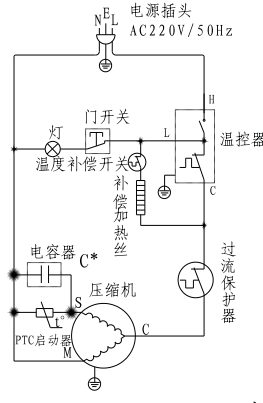
运行电容C*为可选件(根据压缩机选配) 电气原理图
