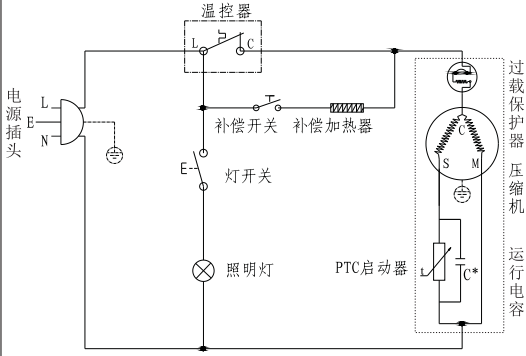
运行电容C*为可选项(根据压缩机选配) 电气原理图
