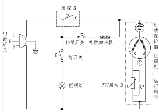
运行电容C*为可选件(根据压缩机选配) 电气原理图
