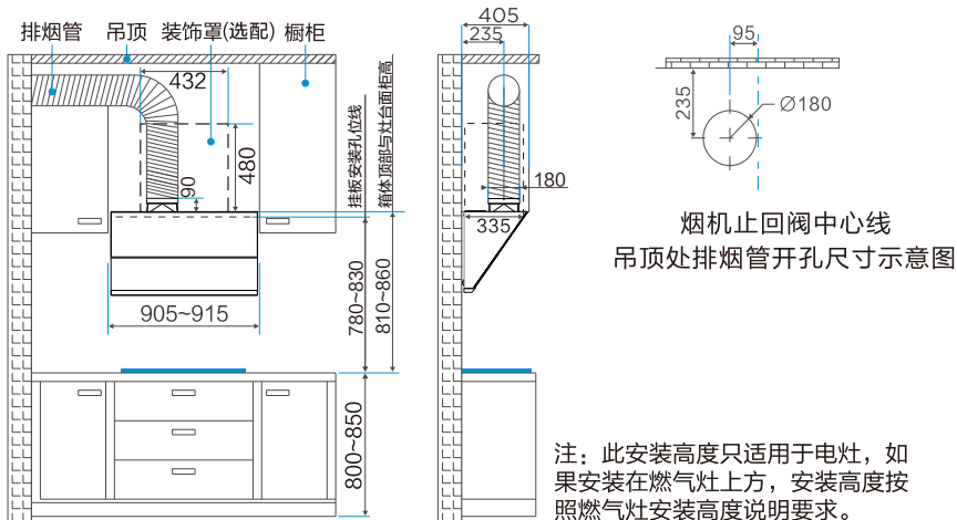
排烟管走橱柜安装示意图
