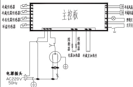
电气原理图
