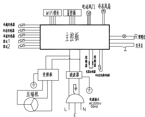
电气原理图
