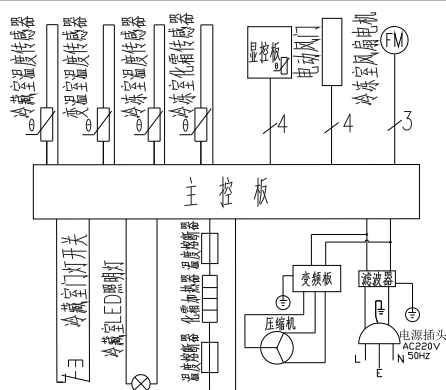
运行电容C*为可选件（根据压缩机选配） 电气原理图
