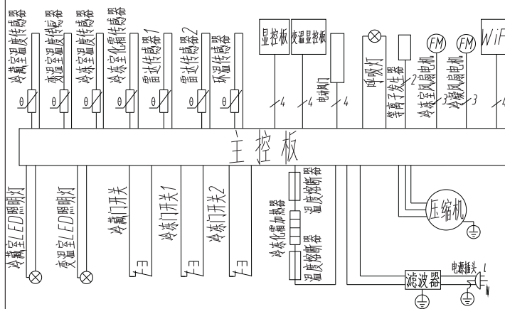
电气原理图
