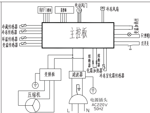
运行电容C*为可选件（根据压缩机选配） 电气原理图
