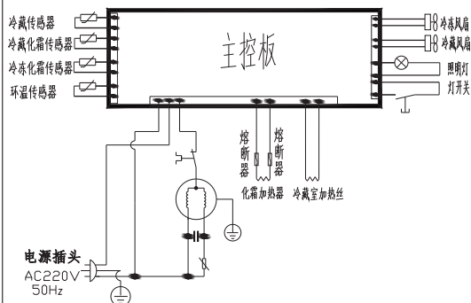
电气原理图
