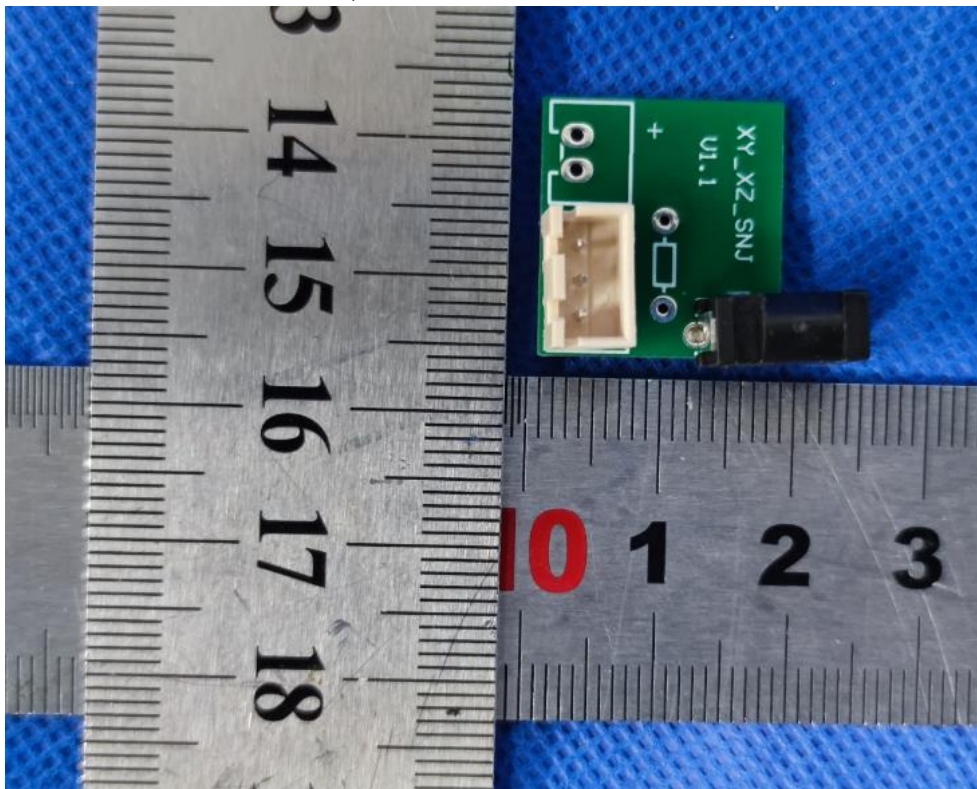
主检型号 X-TSN2701 输入插座 PCB 正面
