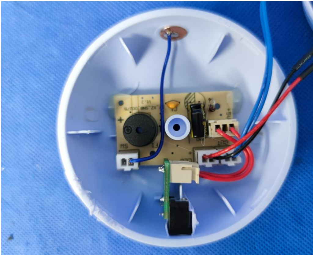
主检型号 X-TSN2701 内部结构
