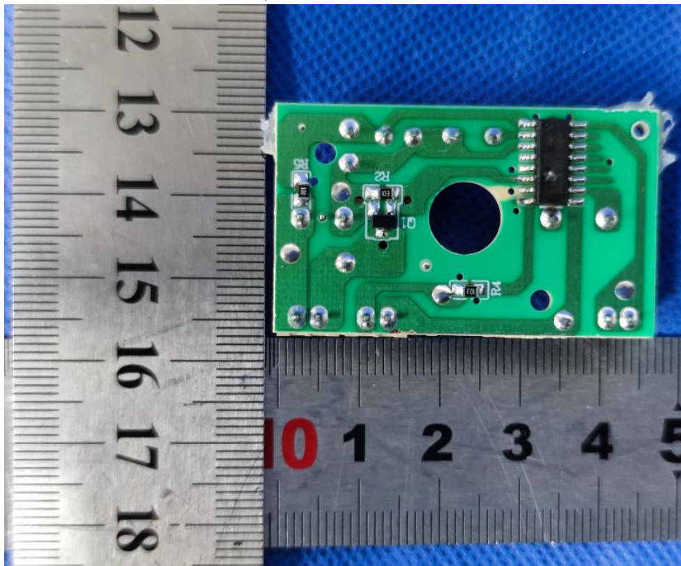
主检型号 X-TSN2701 电源 PCB 反面
