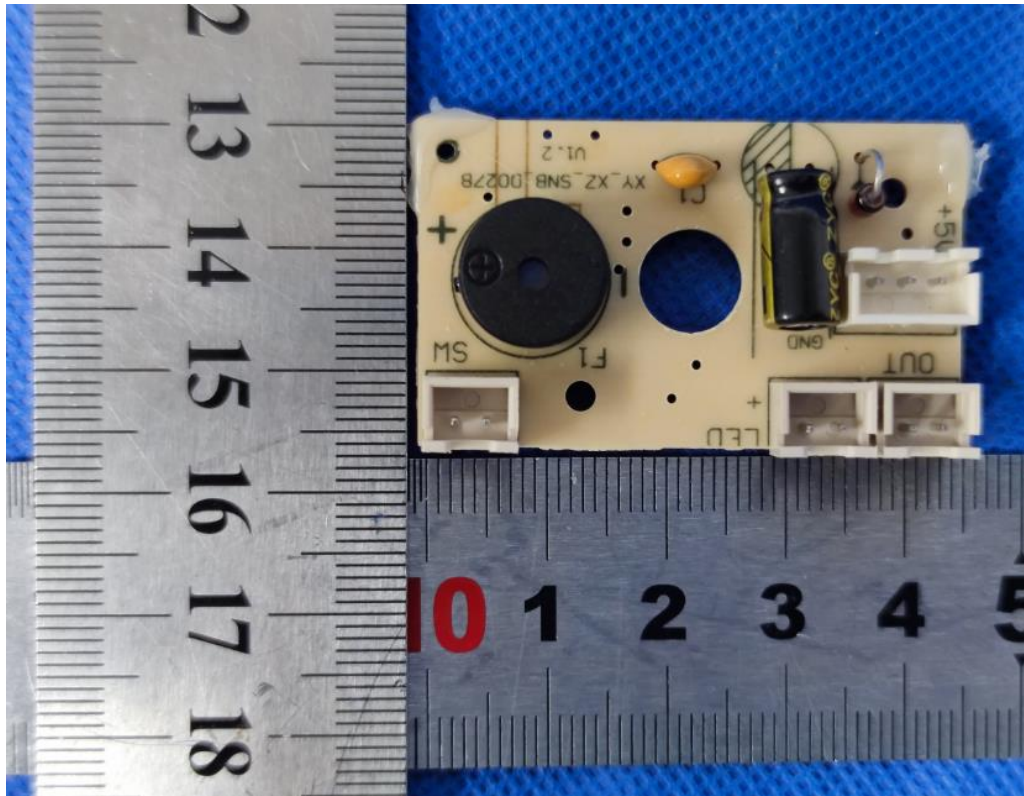
主检型号 X-TSN2701 电源 PCB 正面
