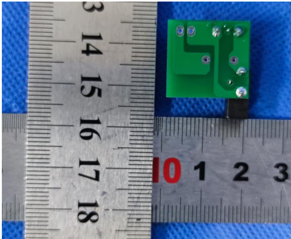
主检型号 X-TSN2701 输入插座 PCB 背面
