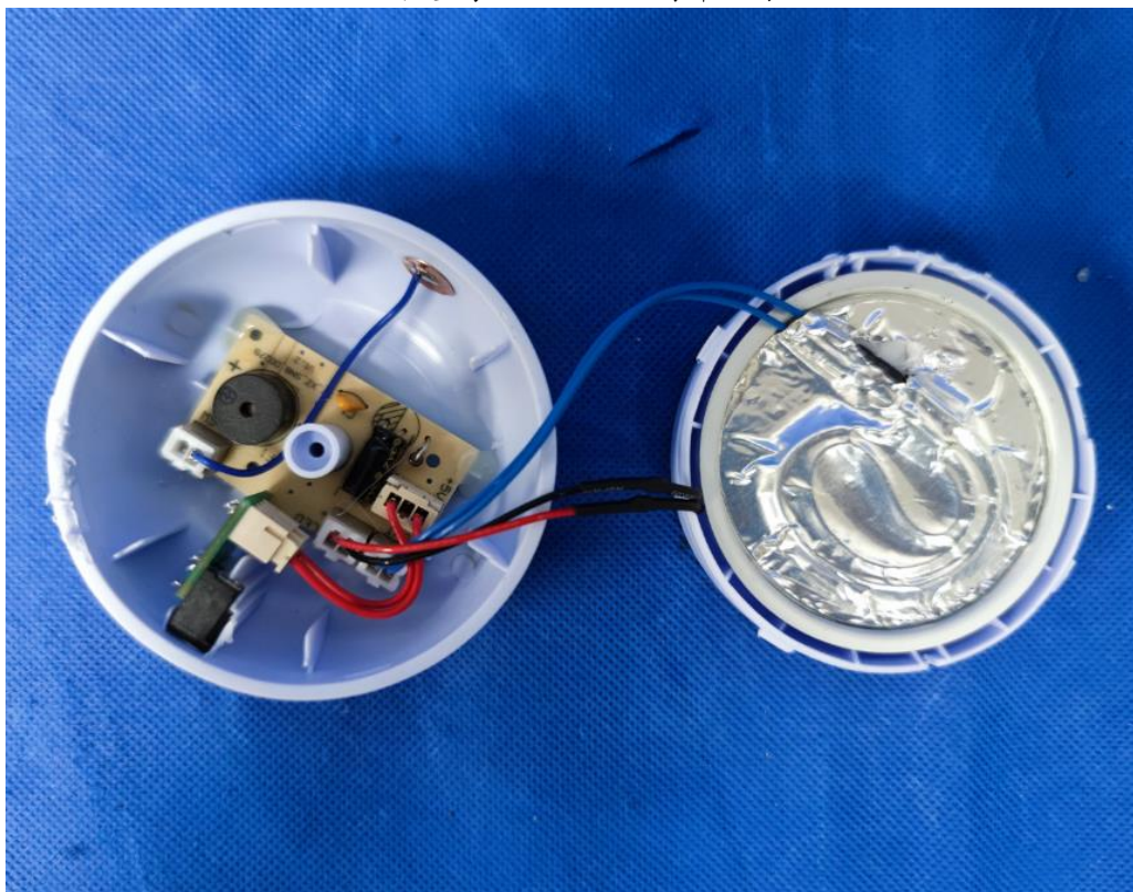
主检型号 X-TSN2701 内部结构
