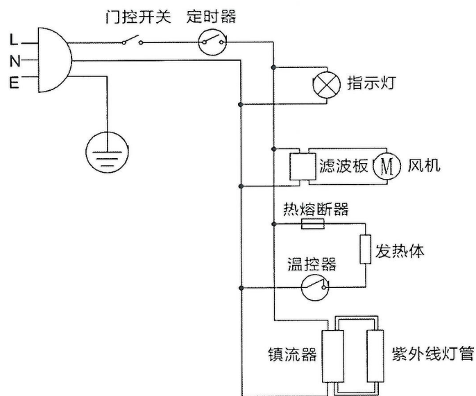
电气原理图
