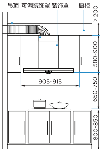
排风管走橱柜安装示意图
