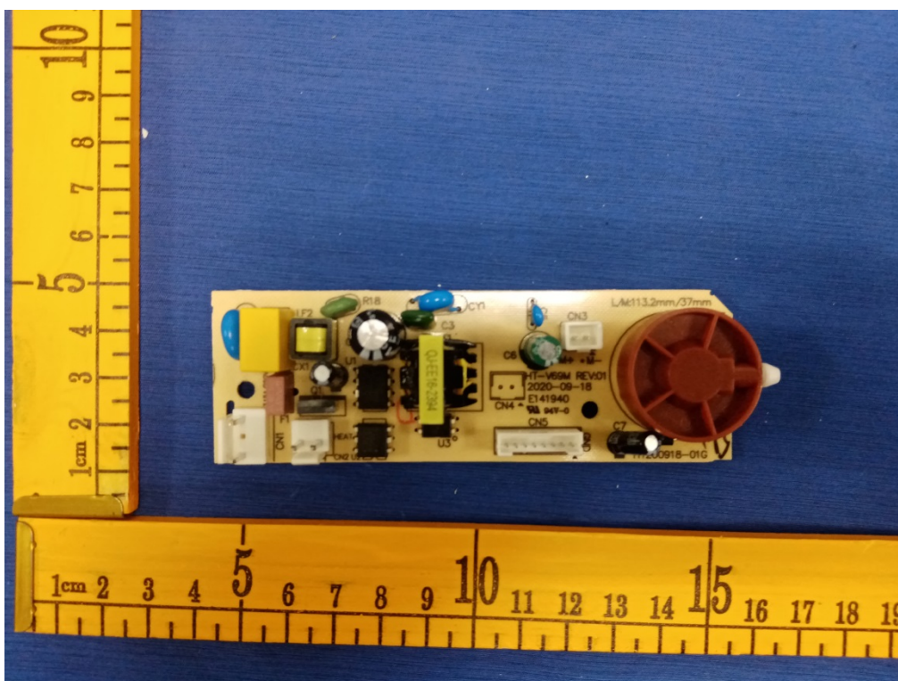
内部结构
