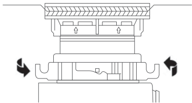
按图示方向锁紧法兰紧固卡环
