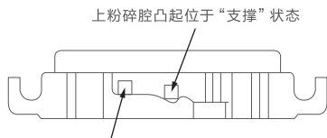
法兰紧固卡环锁紧示意图
