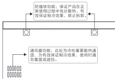
SD/SC-336HKMA产品背部示意图
