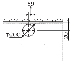
烟机整机中心线 吊顶处排烟管开孔尺寸示意图
