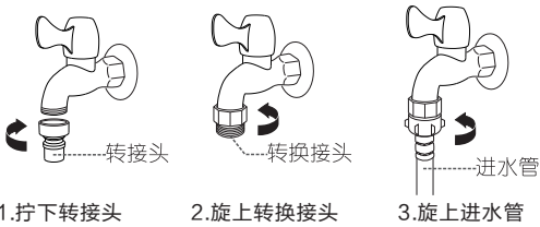
4分水龙头连接
