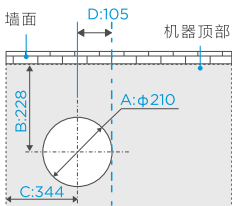
烟机整机中心线
