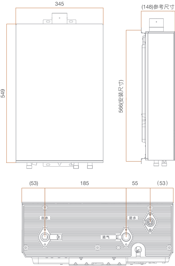
外型尺寸图
