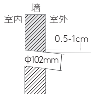
安装选配新风管（内径35/53mm） 需要将墙孔直径扩大到102mm
