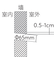
安装标配新风管（内径30mm）， 要求墙孔直径不小于65mm
