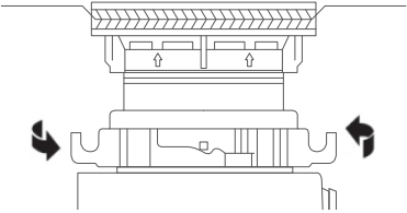
按图示方向锁紧法兰紧固卡环
