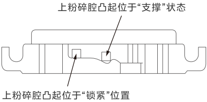
法兰紧固卡环锁紧示意图
