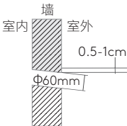
安装标配新风管（内径30mm）， 要求墙孔直径不小于60mm
