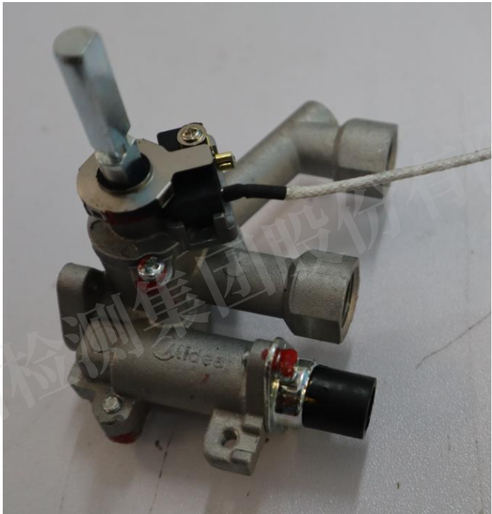
旋塞阀，型号：XSF08-0
