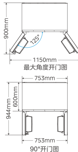
俯视图
