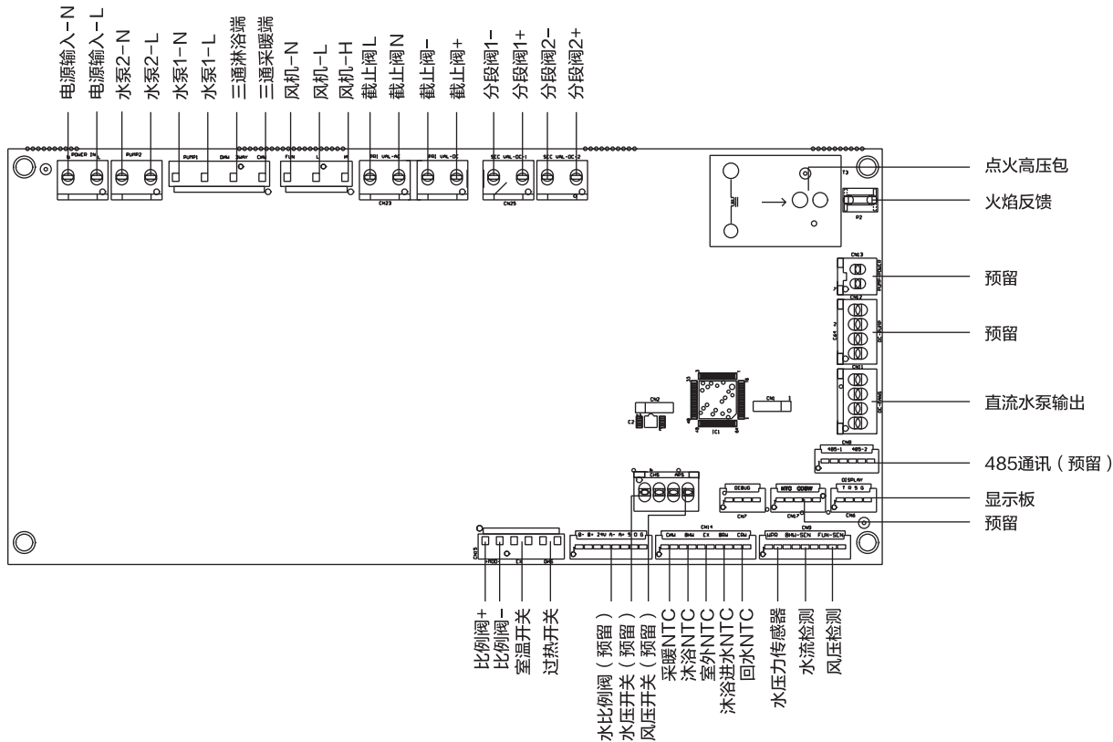
接线示意图
