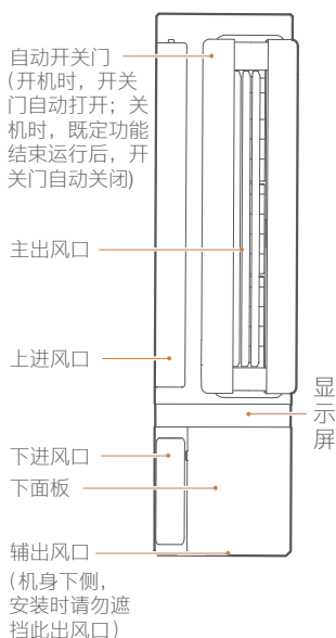
室内机示意图
