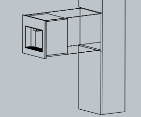
方案二 机器面板四周与柜体层板不搭边安装
