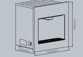
方案一 机器面板四周与柜体层板搭边安装
