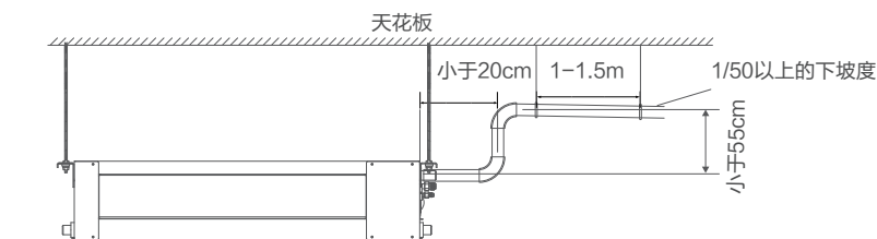
不带水泵机型的安装方式
