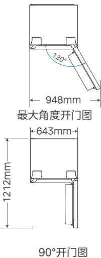
俯视图
