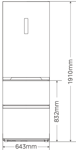
正视图
