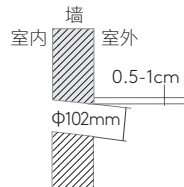
安装选配新风管（内径35/53mm） 需要将墙孔直径扩大到102mm
