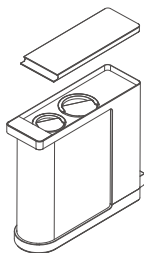
1 打开顶盖装饰件
