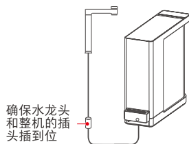
水龙头连整机的电线接线图
