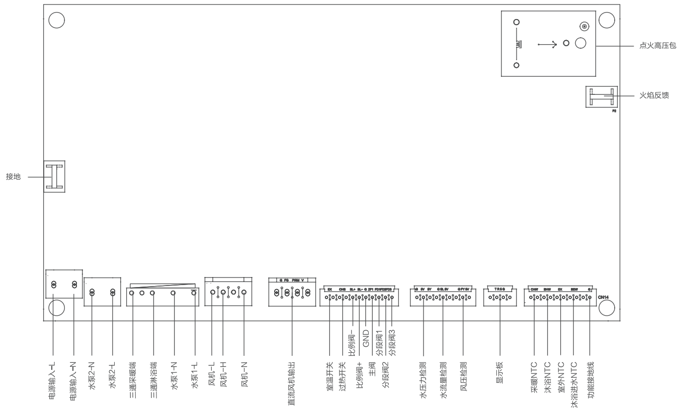
接线示意图
