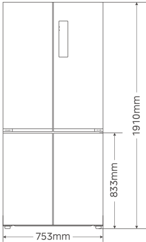
正视图
