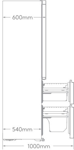
侧视图
