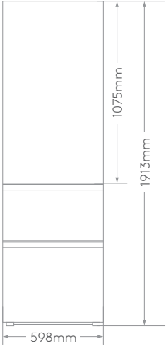
正视图
