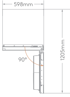
90°开门图
