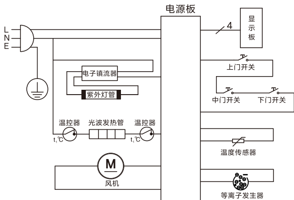
电器原理图
