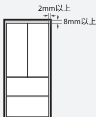
正视图-居中安装
