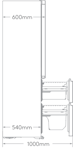
侧视图
