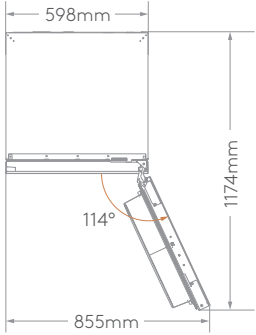
最大角度开门图
