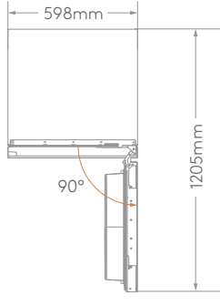
90°开门图
