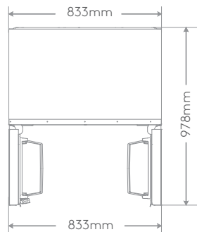
90°开门图
