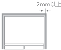
• 俯视图 - 居中安装
