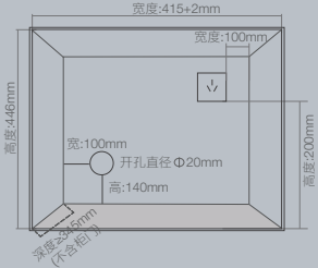
方案一 机器面板四周与柜体层板搭边安装
