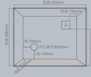
方案二 机器面板四周与柜体层板不搭边安装
