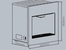
方案一 机器面板四周与柜体层板搭边安装
