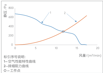
空气性能特性曲线
