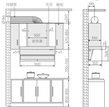
排烟管走橱柜安装示意图
