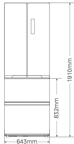
正视图
