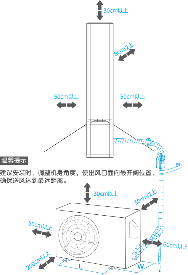
房间空调器使用示意图
