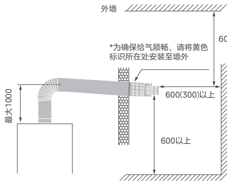
给排气管出口侧面
