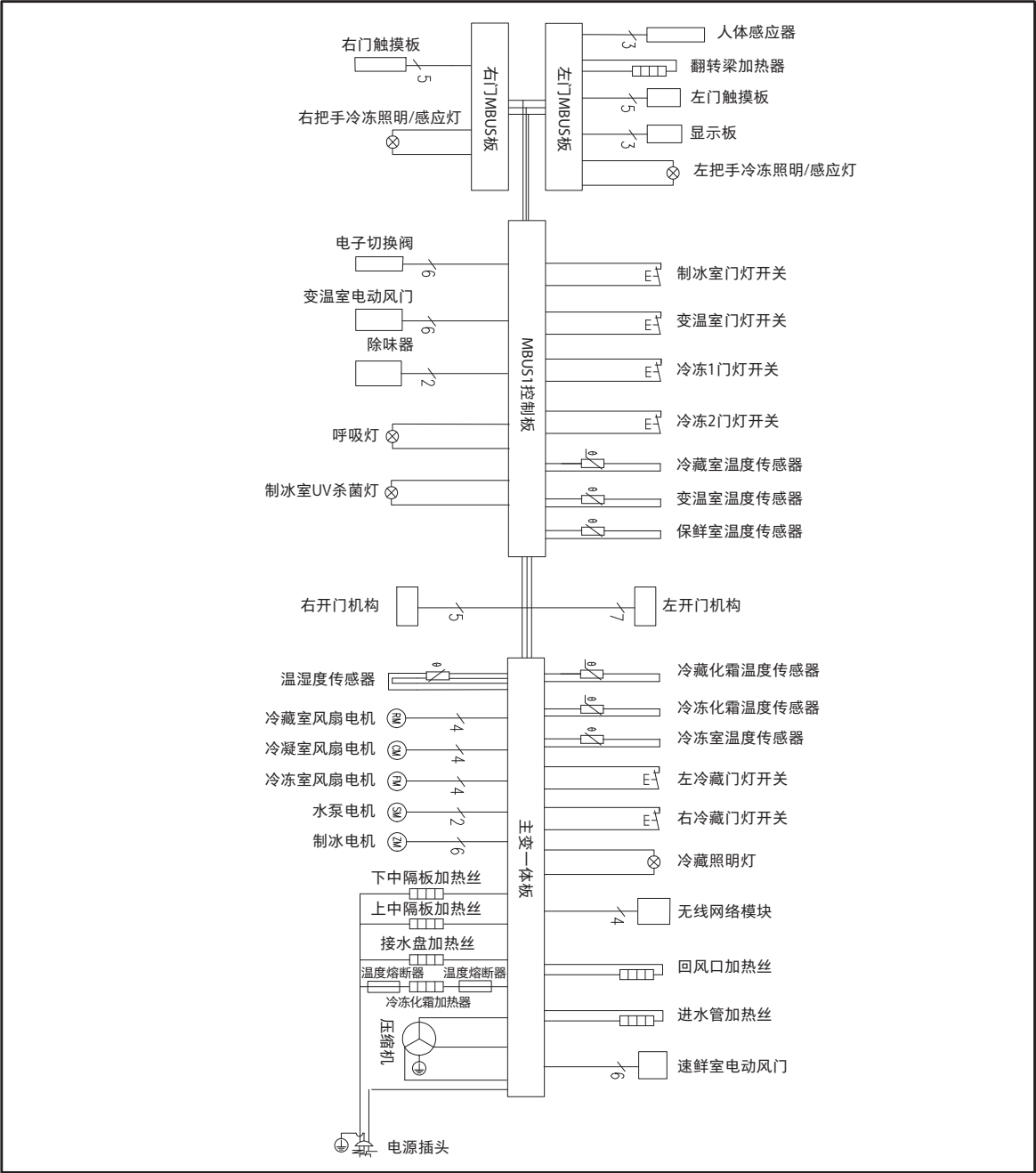
无霜冷藏冷冻箱电器原理图
