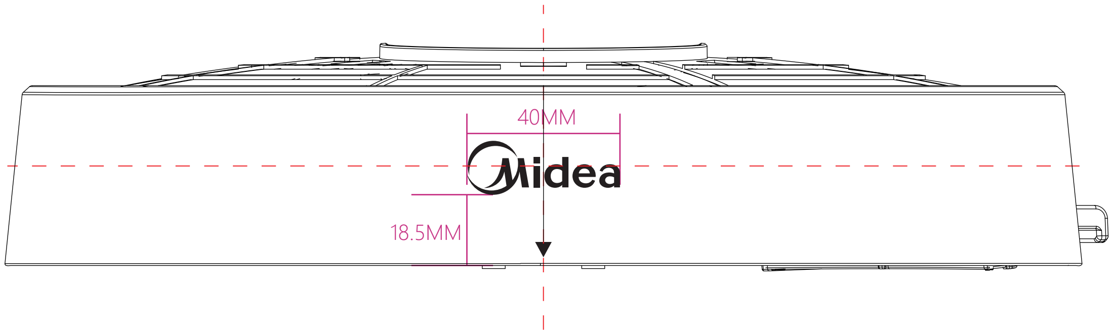
上盖logo标识位置
