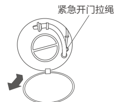
断电情况下，打开过滤器门
