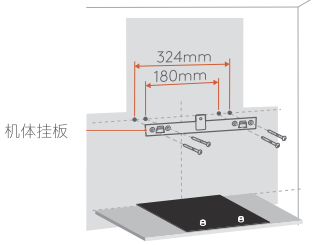
短挂板打孔尺寸
