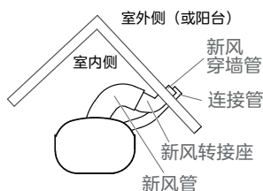
左出管安装示意：
