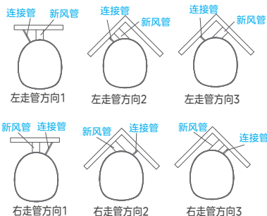
俯视图 走管方向及出管位置
