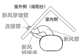
右出管安装示意：
