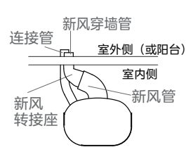
直出管安装示意：
