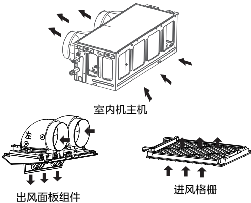
室内机示意图
