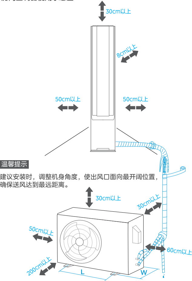
房间空调器使用示意图
