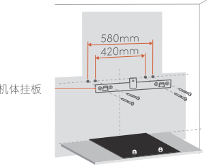
长挂板打孔尺寸
