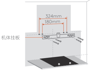
短挂板打孔尺寸
