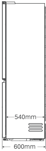
侧视图
