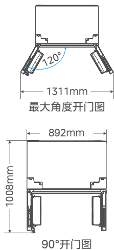
俯视图
