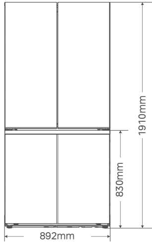
正视图
